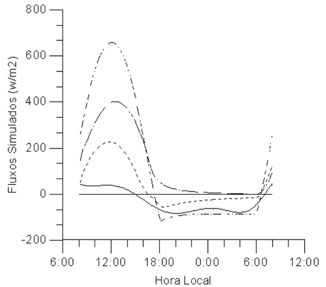
Figura 14 - Evolução temporal simulada em superfície dos fluxos de calor latente (curva tracejada), calor sensível (linha pontilhada), no solo (linha contínua) e saldo de radiação (linha tracejada-pontilhada).
