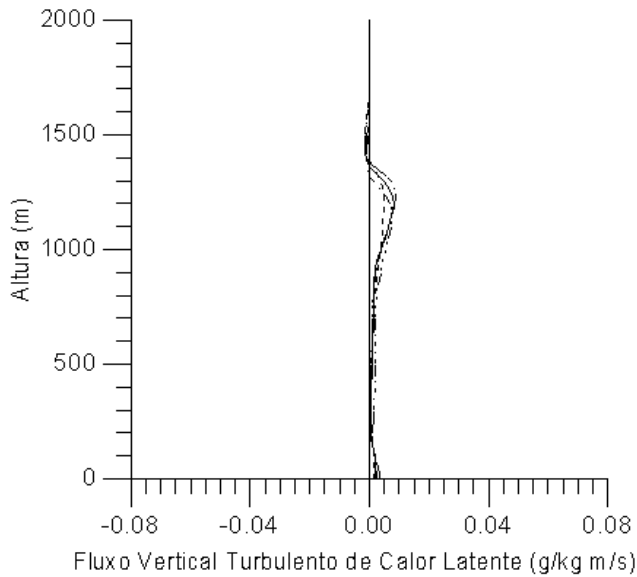
Figura 12 - Perfis vertical simulados de fluxo turbulento de calor latente, para 21:00 h (linha tracejada-pontilhada), 00:00 h (linha contínua), 03:00 h (linha tracejada) e 06:00 h (linha pontilhada).
